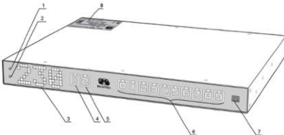
Рисунок 4.1.1. Лицевая панель RPCM 1502 (16A) и RPCM 1532 (32A).
