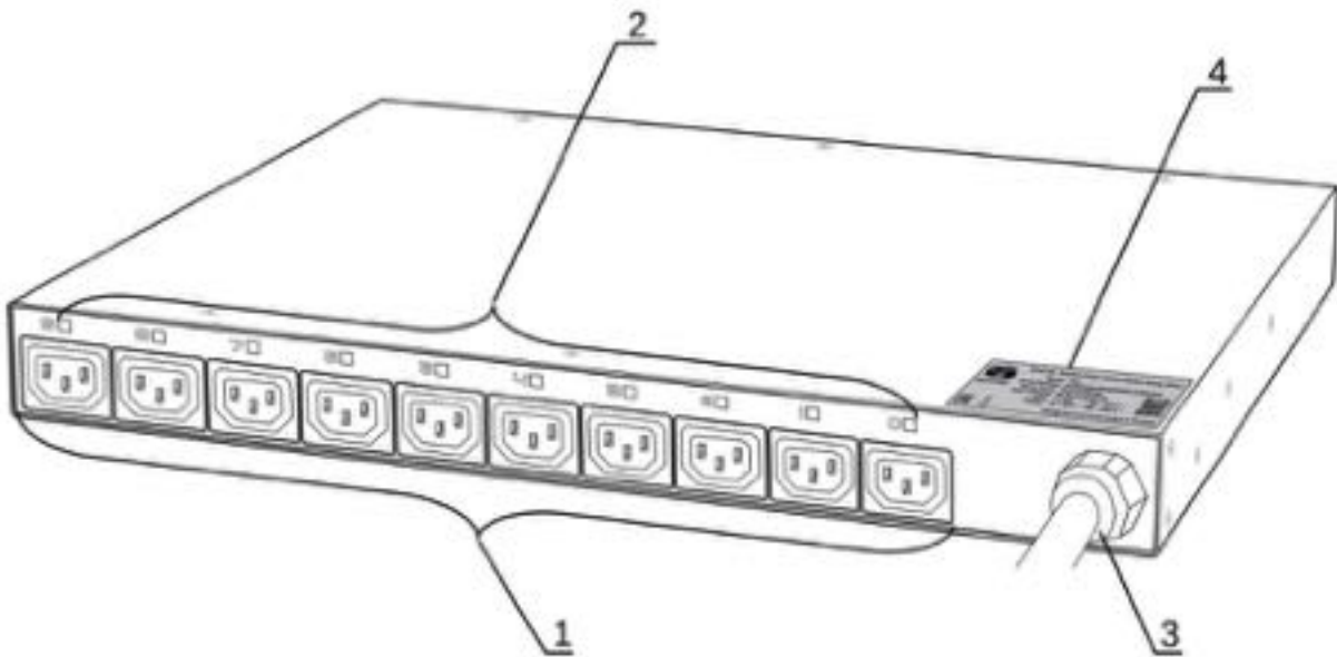
Рисунок 4.1.5. Задняя сторона РСМ ME 1563 (63A)
