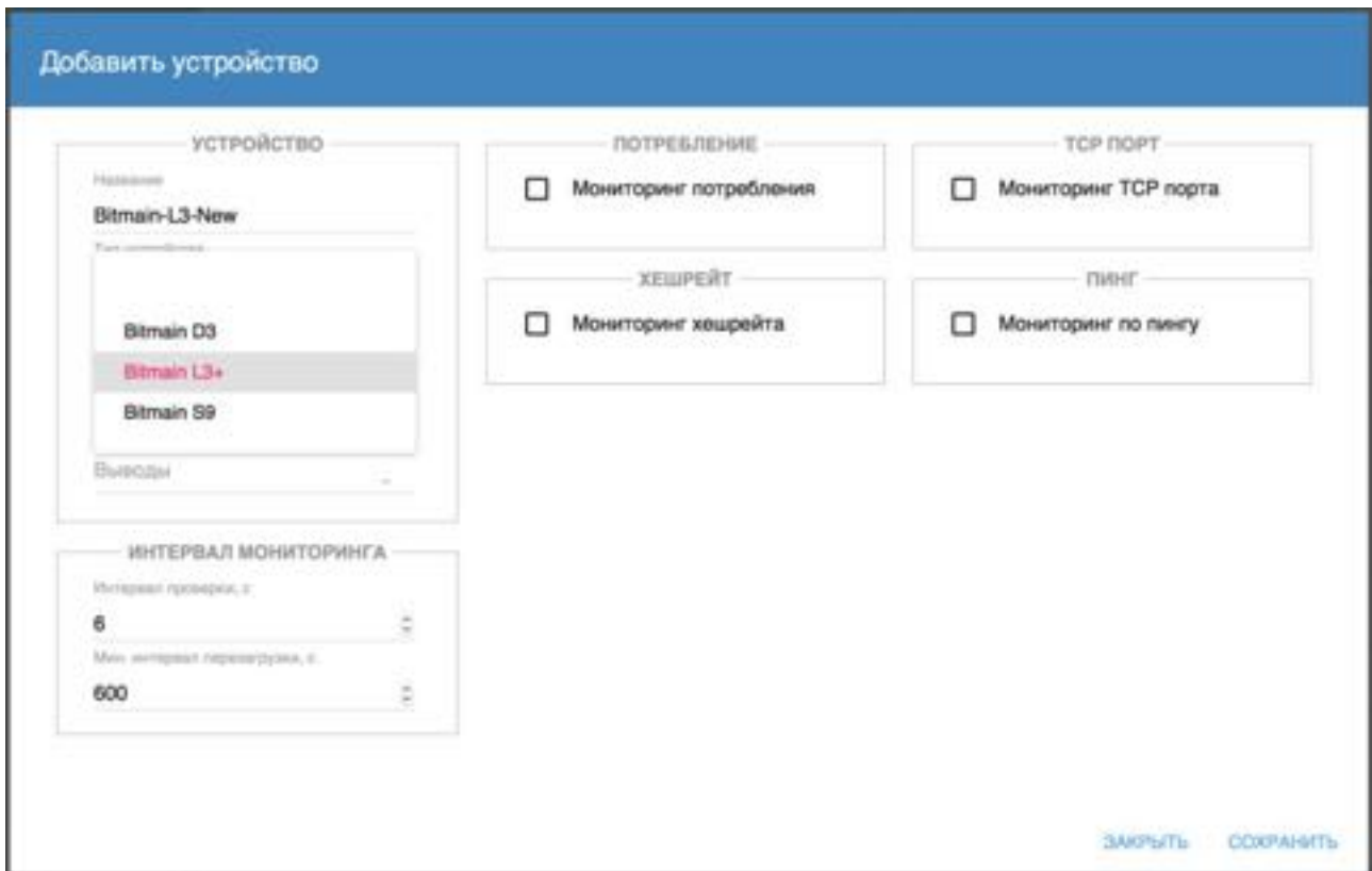
Рисунок 4.11.13. Всплывающее окно "Добавить устройство" с вызванным меню Тип устройства.
