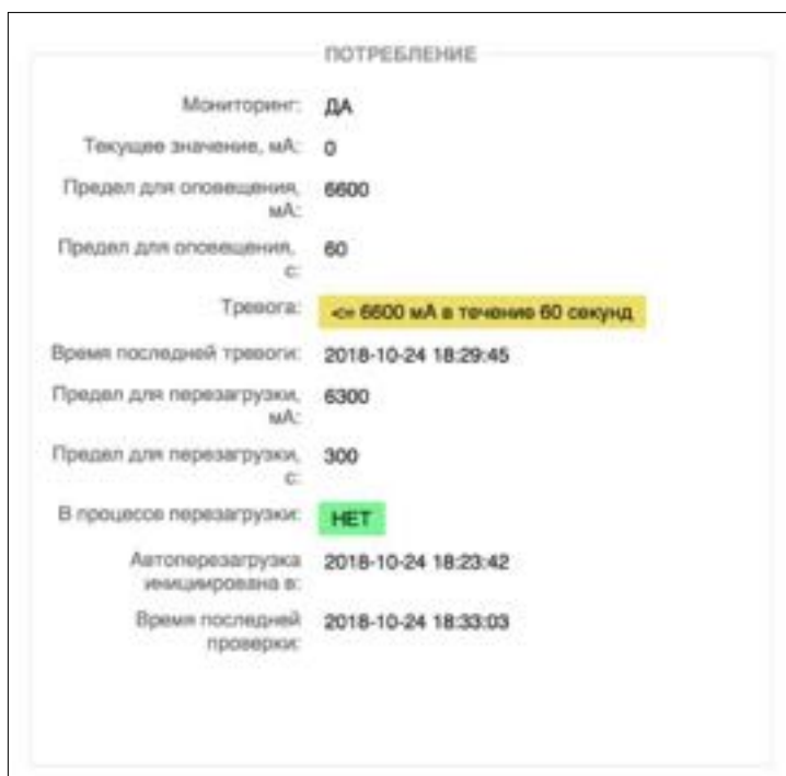
Рисунок 4.11.5. Раздел "Автоматизация" — подраздел "ПОТРЕБЛЕНИЕ".
