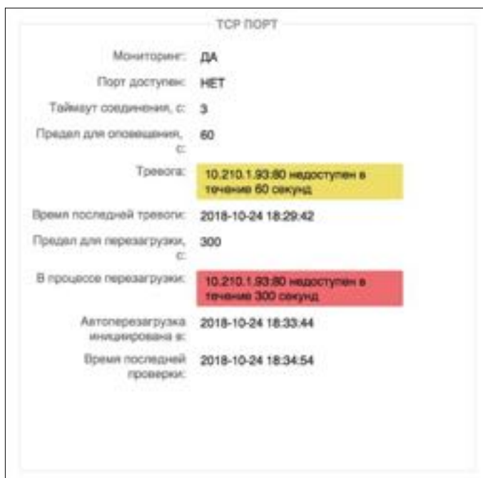
Рисунок 4.11.8. Раздел "Автоматизация" — подраздел "TCP порт".
