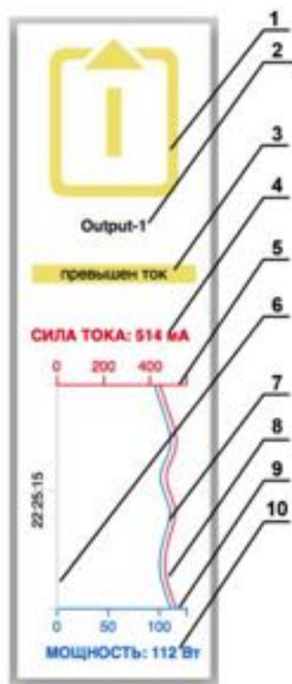
Рисунок 4.2.6. Блок информации о состоянии вывода в режиме просмотра (View Mode).
