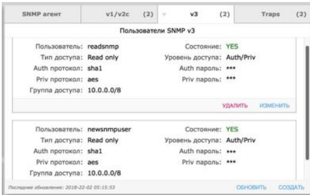
Рисунок 4.6.31. Область управления SNMP, вкладка "SNMP v3 Users". Новая запись пользователя SNMPv3 "newsnmpuser" создана.
