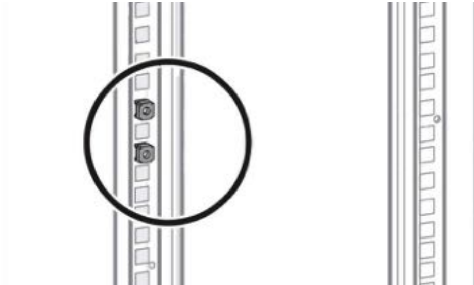
Рисунок 2.2.1. Установка клетевых стоечных гаек в монтажной стойке.
