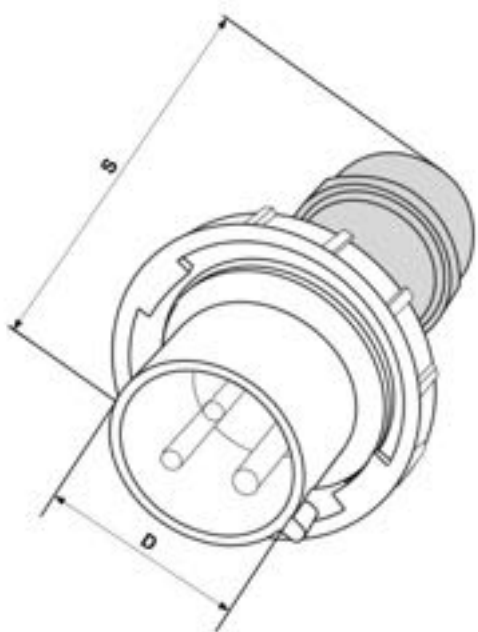
Рисунок 2.2.5. Разъём 2P+PE 32А 250V, установленных на РСМ 32А (1532).
