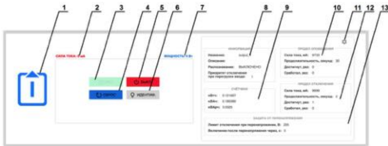
Рисунок 4.5.6. Управление состоянием выводов в режиме управления (Control mode).
