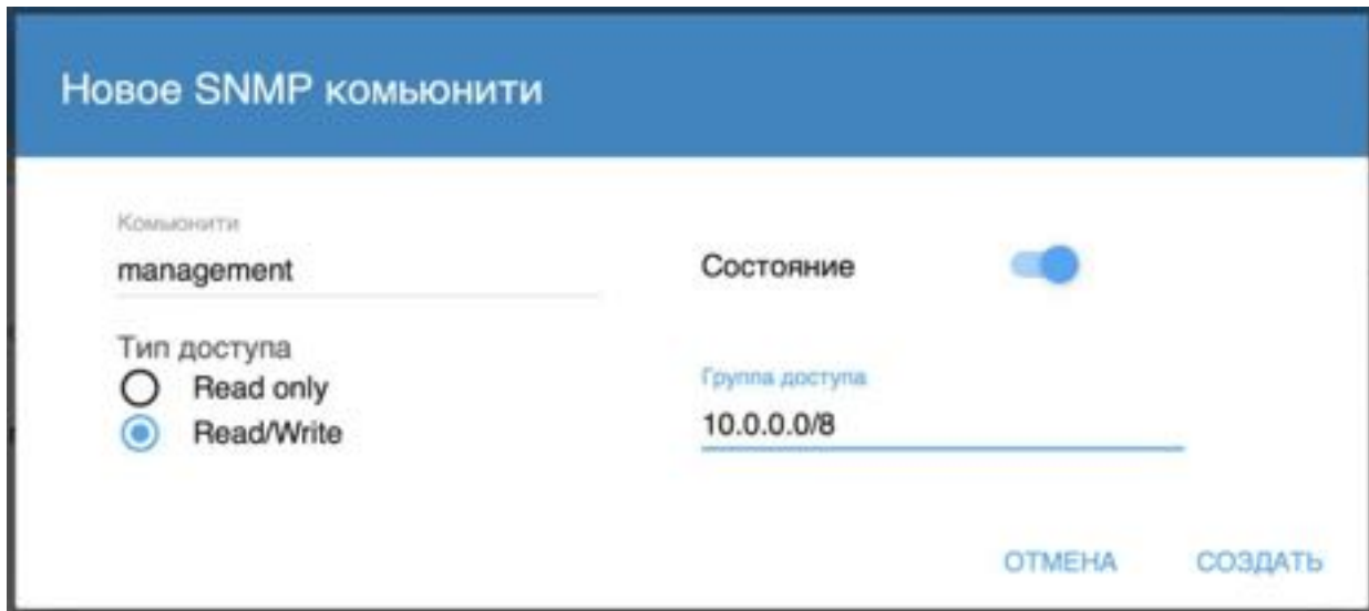
Рисунок 4.6.25. Всплывающее окно "Новое SNMP комьюнити". Переключатель "Состояние" — ON
