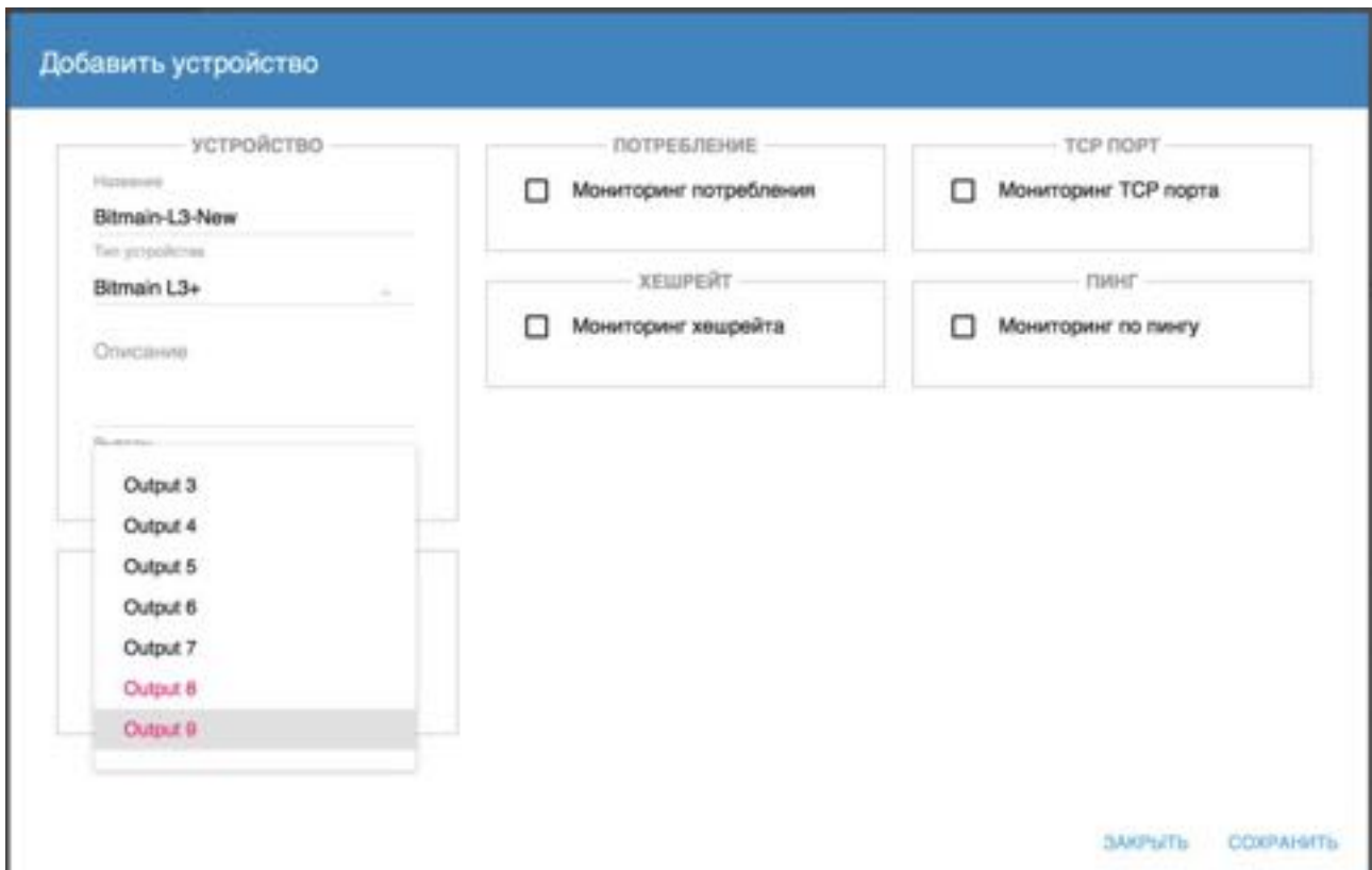
Рисунок 4.11.14. Выбор выводов Output 8 и Output 9 в окне "Добавить устройство".
